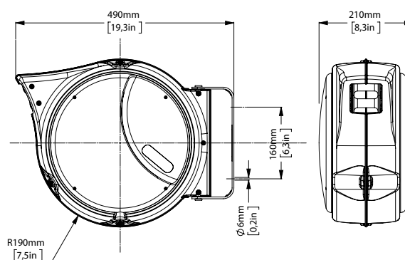
dimensioni AM85
