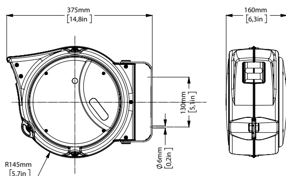
dimensioni AM80
